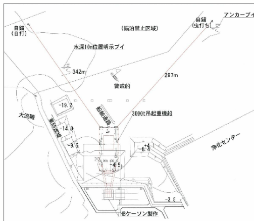
ハイブリッドケーソン吊上配置図
