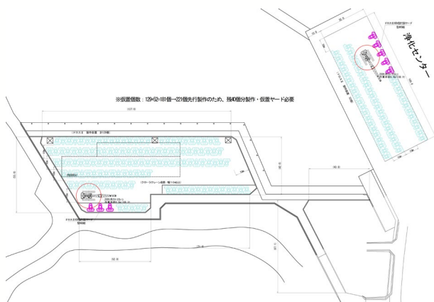
年次ヤード使用状況図（16年目）
