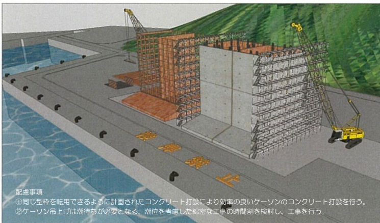
ハイブリッドケーソン製作イメージ図
